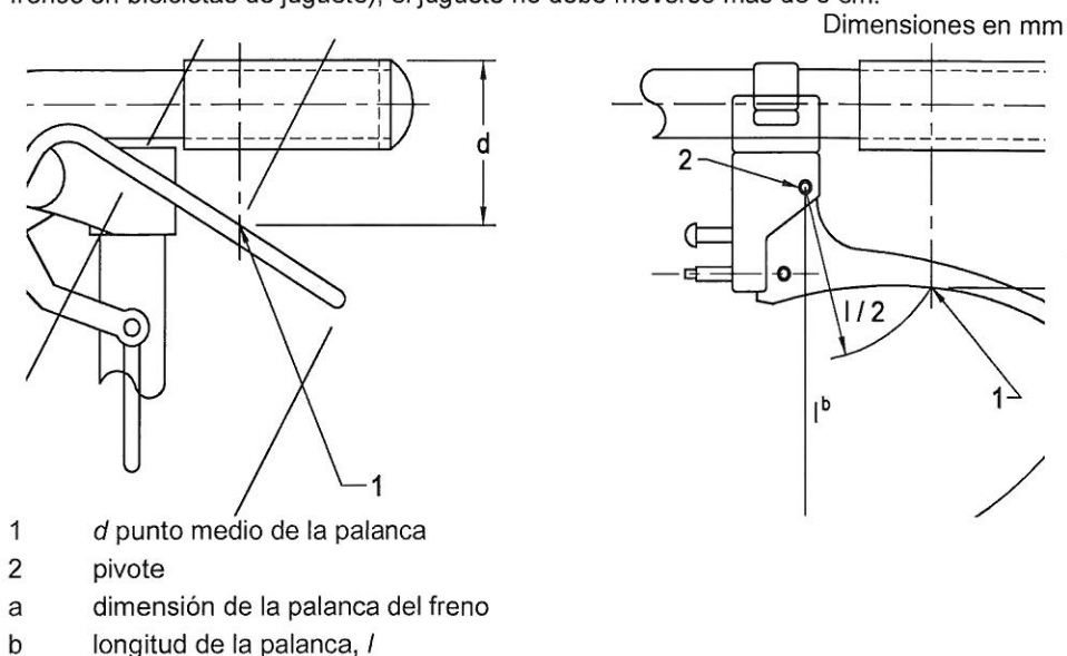
Figura 12. Dimensiones de la palanca del freno manual
