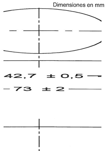
Figura 15. Plantilla complementaria de ensayo B
