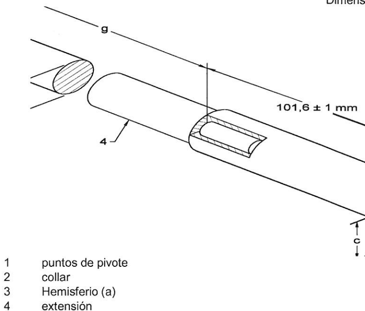
Figura 17. Sonda de accesibilidad
