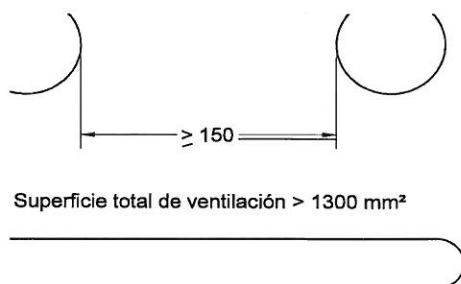
Figura 11. Ejemplo de área de ventilación alternativa
